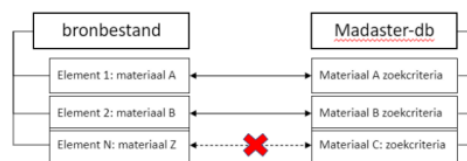
Figuur 66 Matchen van element (uit bronbestand) aan toegevoegd in Madaster-database (conceptweergave).
